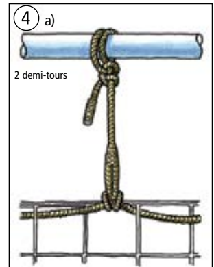
4 a) 2 demi-tours Suspension du filet par entrelacement et nouage du câble de suspension sur l'élément de support Câble de suspension à un brin L (Résistance de rupture de câble \geq 30 \text{ kN} )
