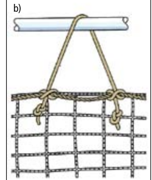
4 b) Câble de suspension à deux brins Z (Résistance de rupture de câble \geq 15 \text{ kN} ) Les câbles sont à protéger contre tout risque de détorsion et ne doivent pas pouvoir être endommagés par des arêtes tranchantes.
